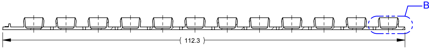
SECTION A-A SCALE: 1.6 : 1
