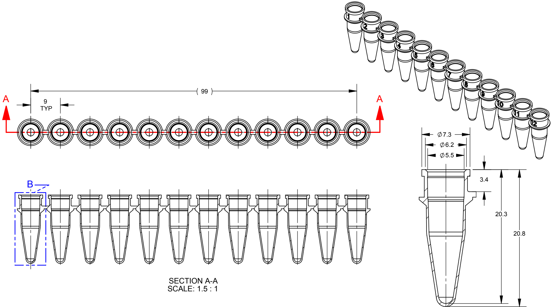
DETAIL B SCALE: 3 : 1
