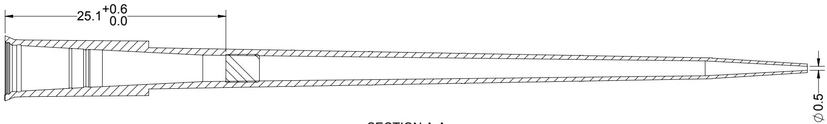
SECTION A-A
